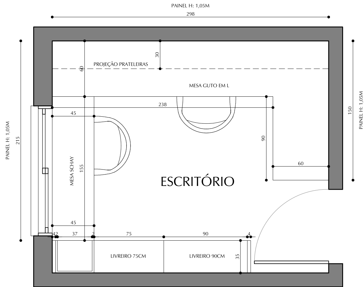
PLANTA BAIXA ESCALA: 1/25
